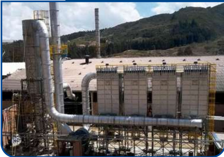
FILTROS DE MANGAS PARA GASES
